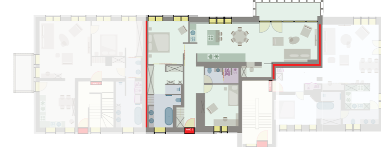
GRUNDRISS EG | WOHNUNGEN 1-3
